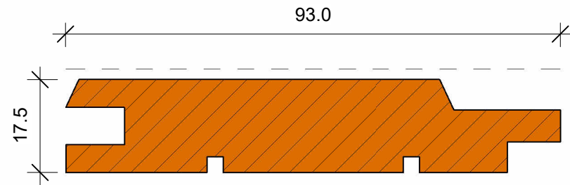
6601-3 CT TGV BÅND 22x100 1:1
