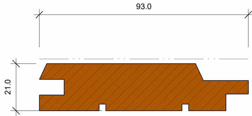
7201-1 TF TGV GLAT 25x100 1:1
