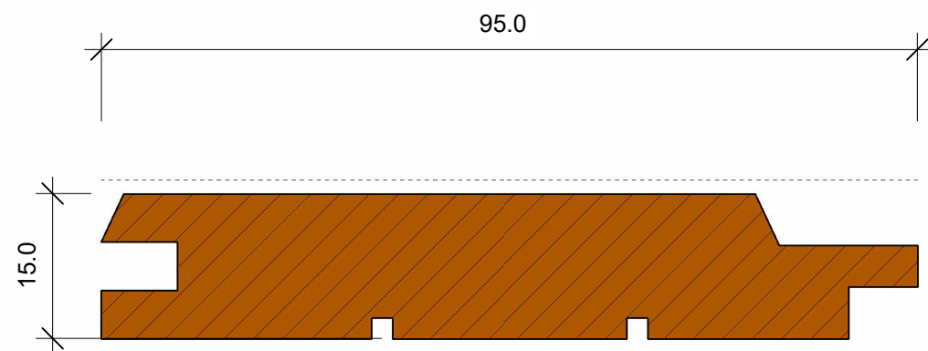
2950-1 TGV 19x100 1:1
